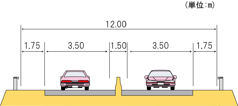
＜今回開通区間の標準横断面図＞
