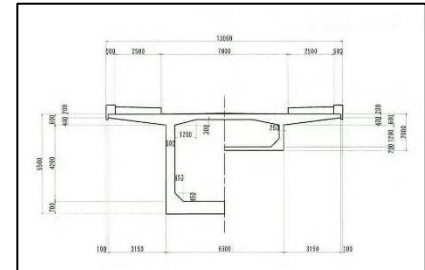
標準断面図
