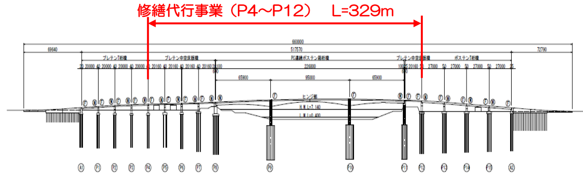
側面図
