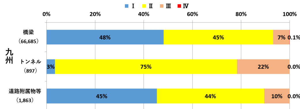
2巡目点検の点検結果(九州版)
