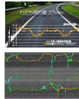
走行しながら測定を行い、ひび割れ率、わだち掘れ率、IRI等を算出
