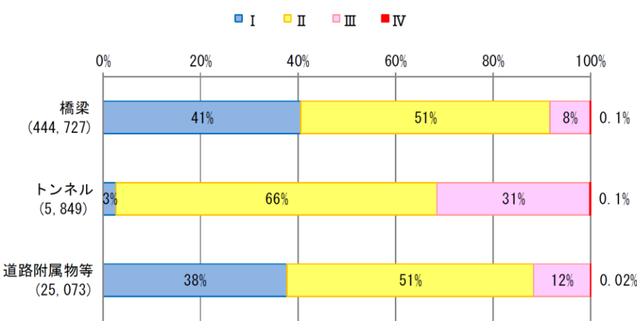
2巡目(2019～2021年度)の点検結果
