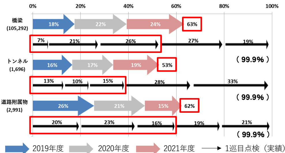
2021年度の点検実施状況(九州版)
