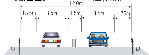
《断面図》
